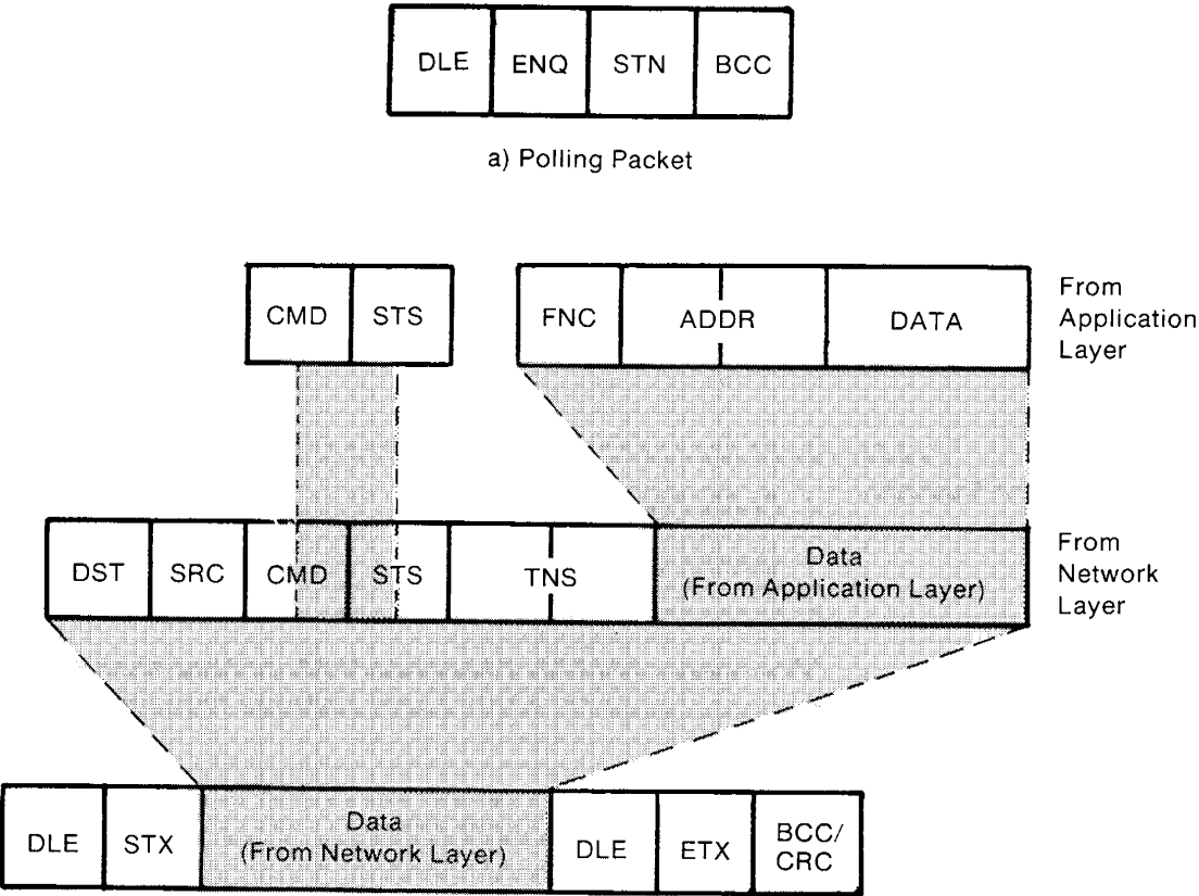
b) Slave Message Link Packet
