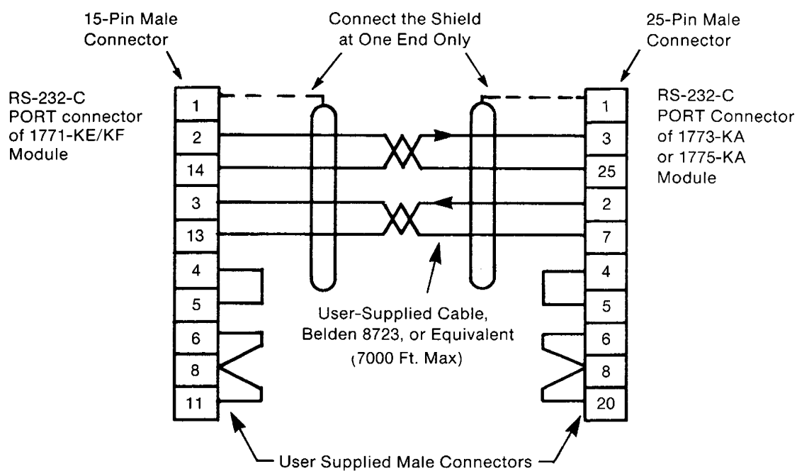
b) Wiring Diagram
