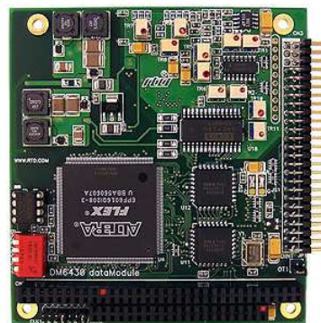
DM6430 dataModule
