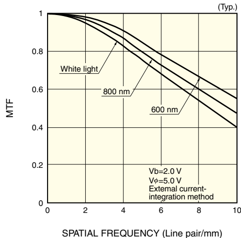
Figure 4-15 MTF (S3901-512Q)
