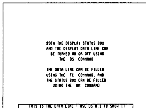
Fig. 20. Display Data Line Box
