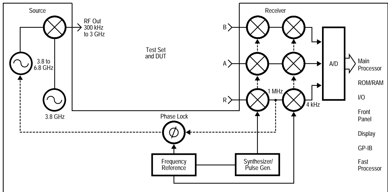
Agilent 8702E Option 8702E-011 block diagram
