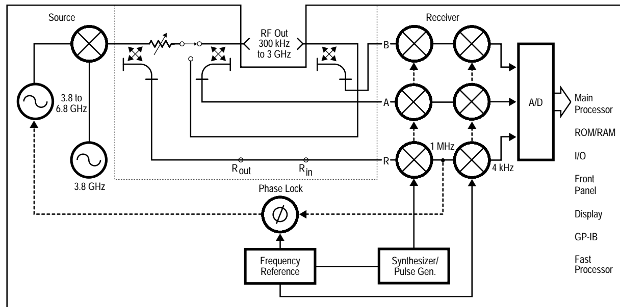
Agilent 8702E block diagram
