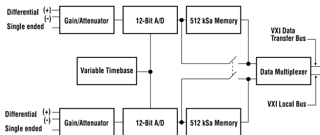
HP E1429B Block Diagram
