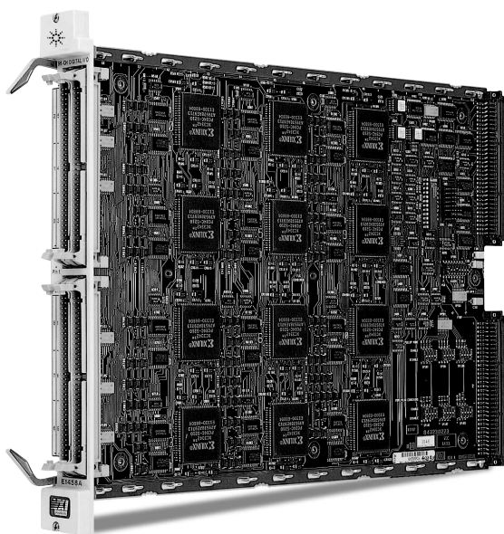
Agilent E1458A
