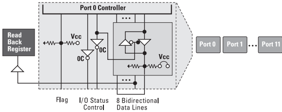
Agilent E1458A Block Diagram
