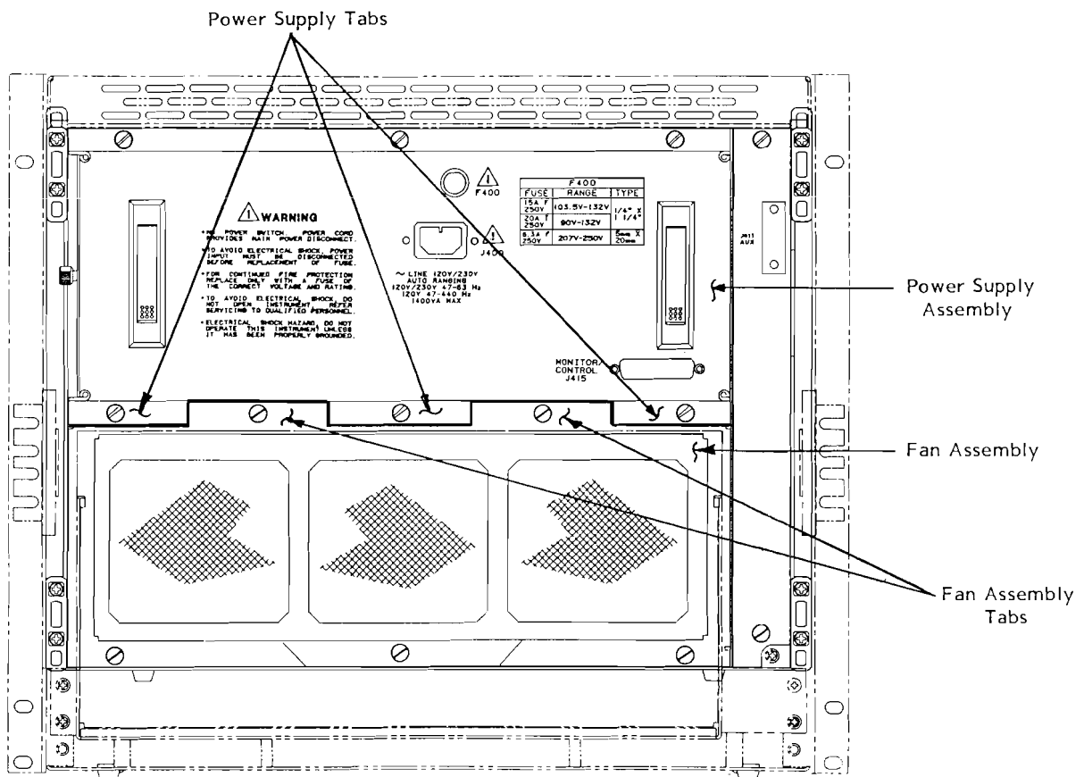
Figure 5-4 Aligning The Module Fan Assembly
