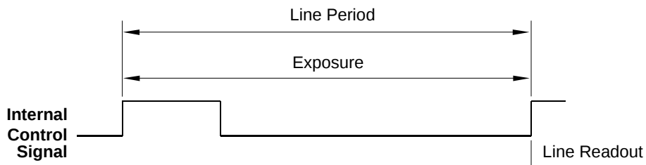
Fig. 30: Free Run, Edge Controlled Mode
