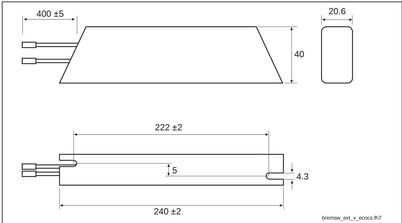
Fig. 10-33: Dimensions
