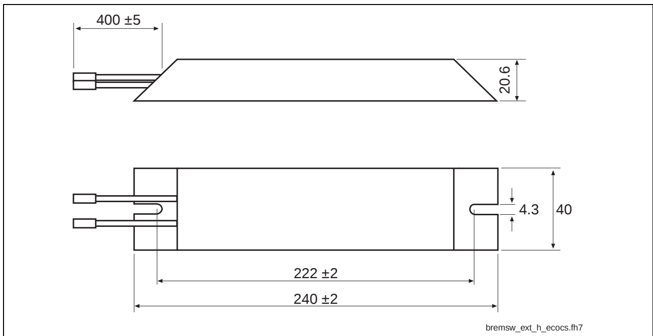
Fig. 10-34: Dimensions
