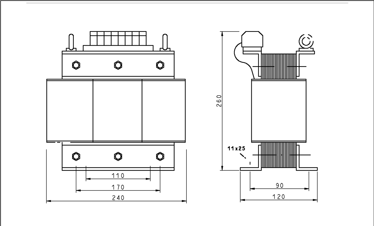
Fig. 10-47: Dimensions
