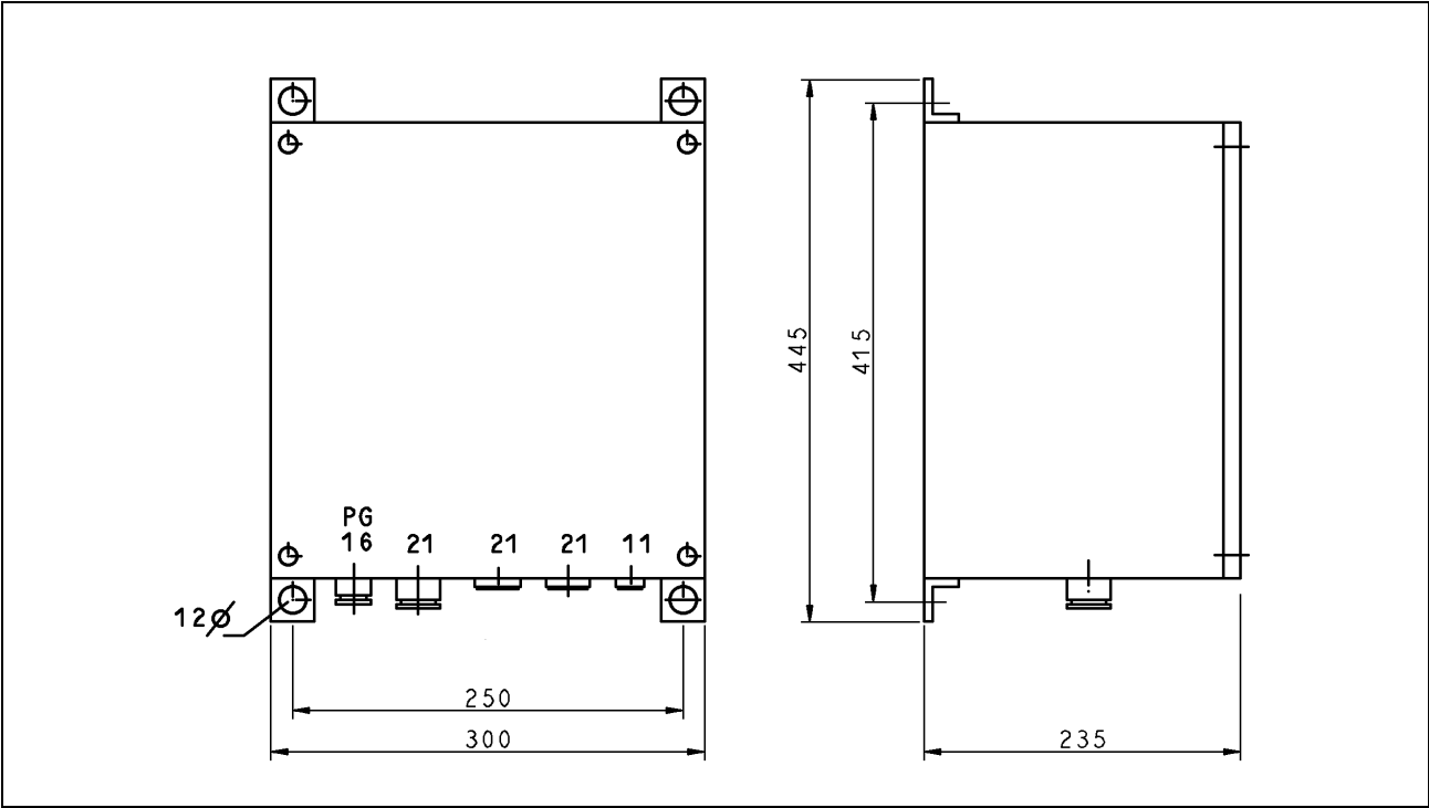
Fig. 10-51: Dimensions
