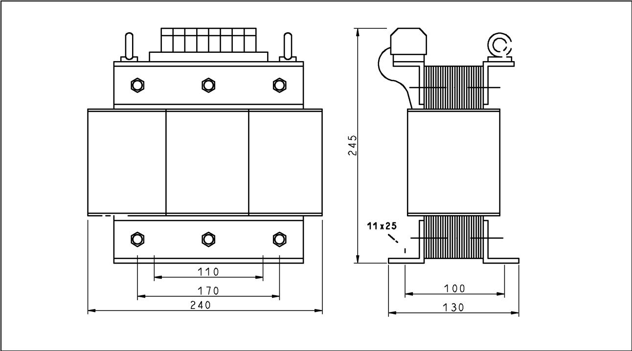
Fig. 10-43: Dimensions
