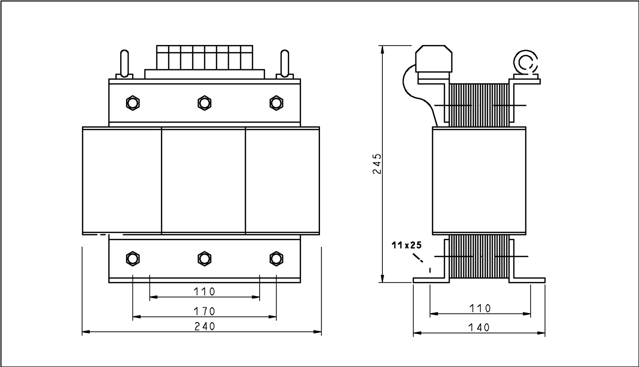
Fig. 10-49: Dimensions
