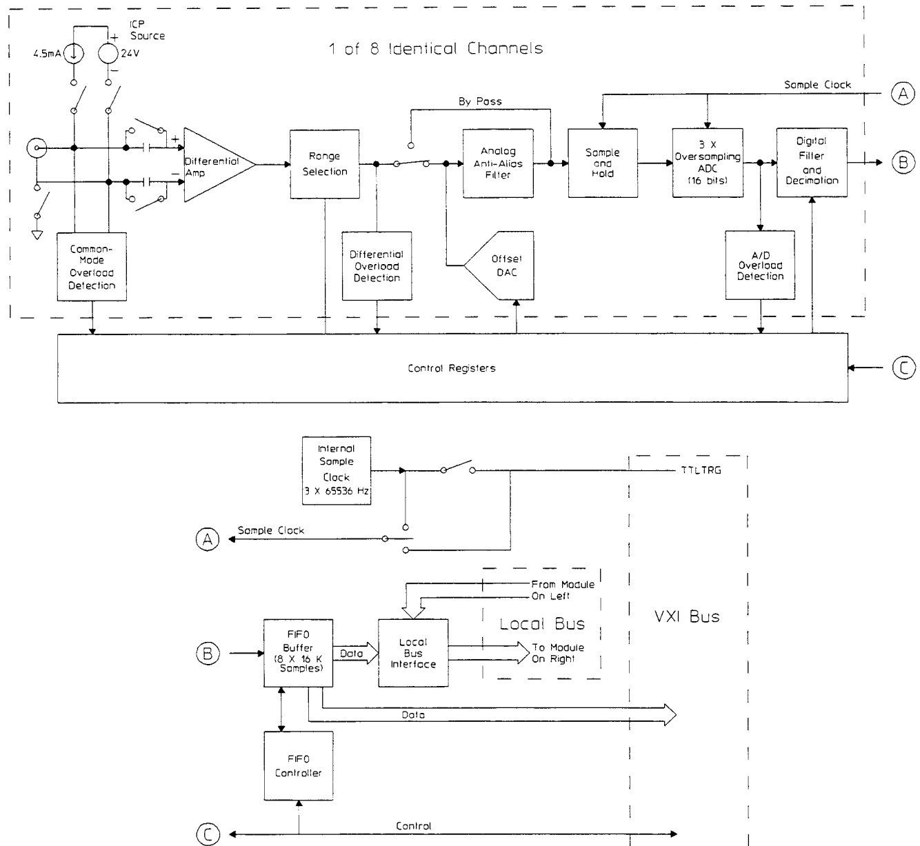
HP E1431A Block Diagram
