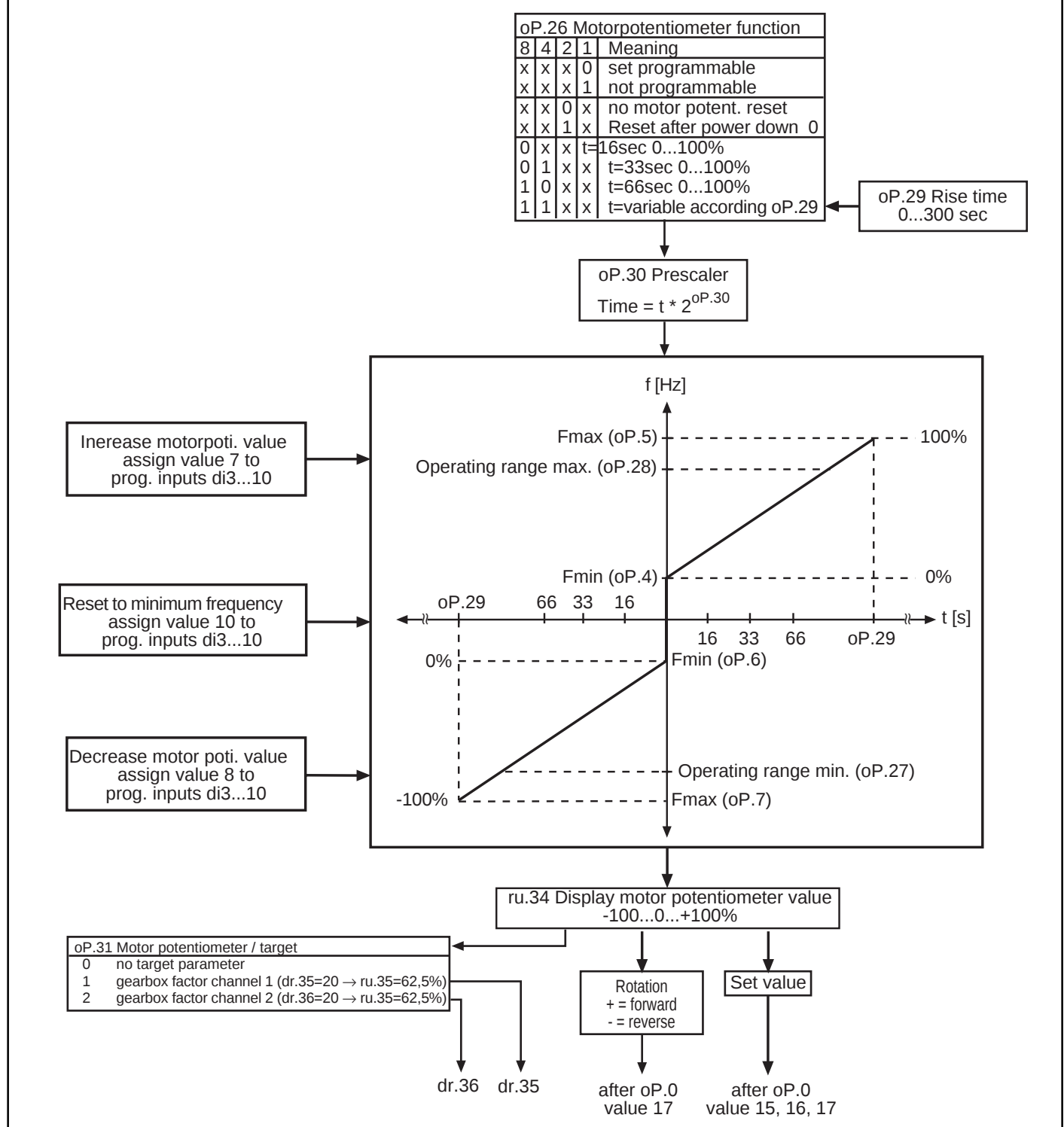
Fig. 6.9.4 Motor Potentiometer Function
