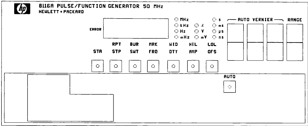
Figure 4-10. Parameter controls
