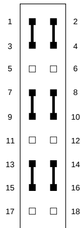
1Mx8 EPROM
