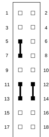
2Kx8 or 8Kx8 EEPROM
