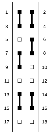
512Kx8 EPROM
