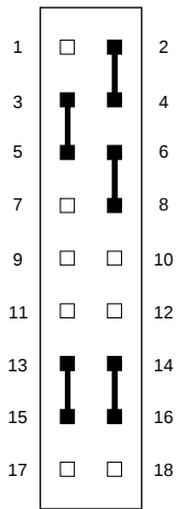
128Kx8 EPROM
