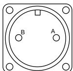
MS3102E14S-9P
