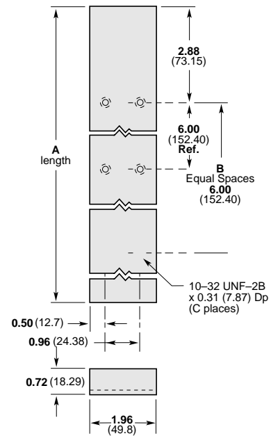
Platen
