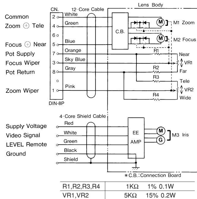
TYPE 2 (DC 12V)
