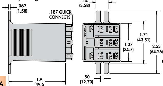
Top Flange - Code C3
