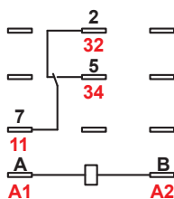
SPDT
