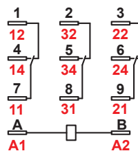
3PDT
