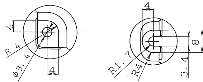
BEZEL/DISPLAY POSITION
