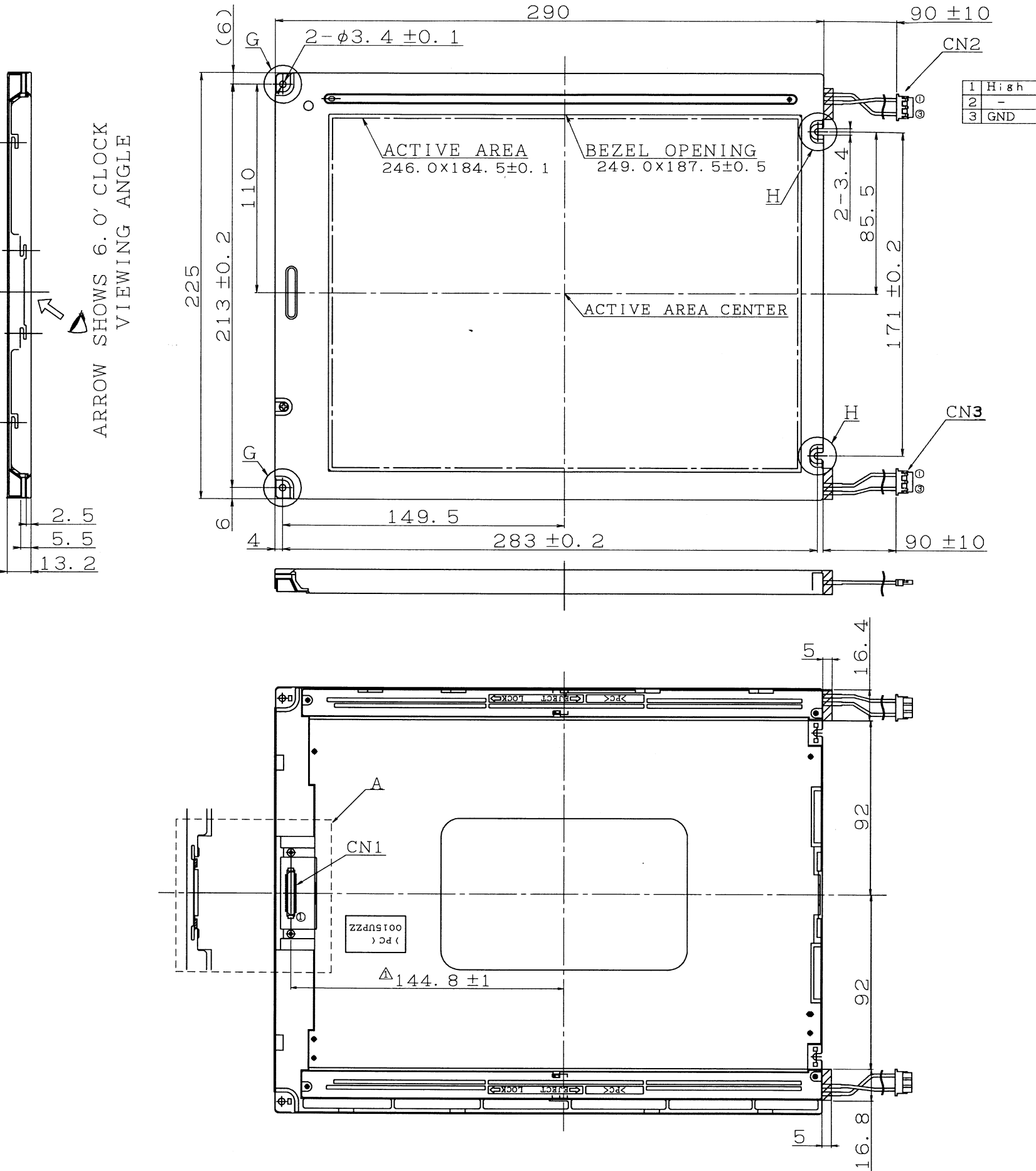
FIG1 LQ121S1DG11 OUTLINE DEMENSIONS
