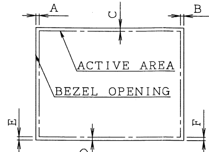
BEZEL/DISPLAY POSITION
