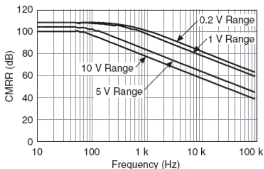
AI <0..79> CMRR
