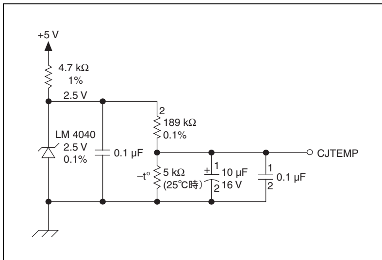
図 4 温度センサ回路図
