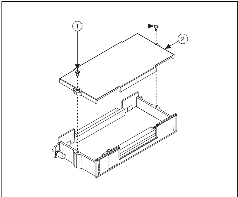
図 1 SCXI-1331 上部カバー
