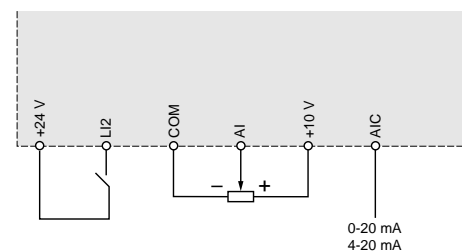
Wiring schematic
